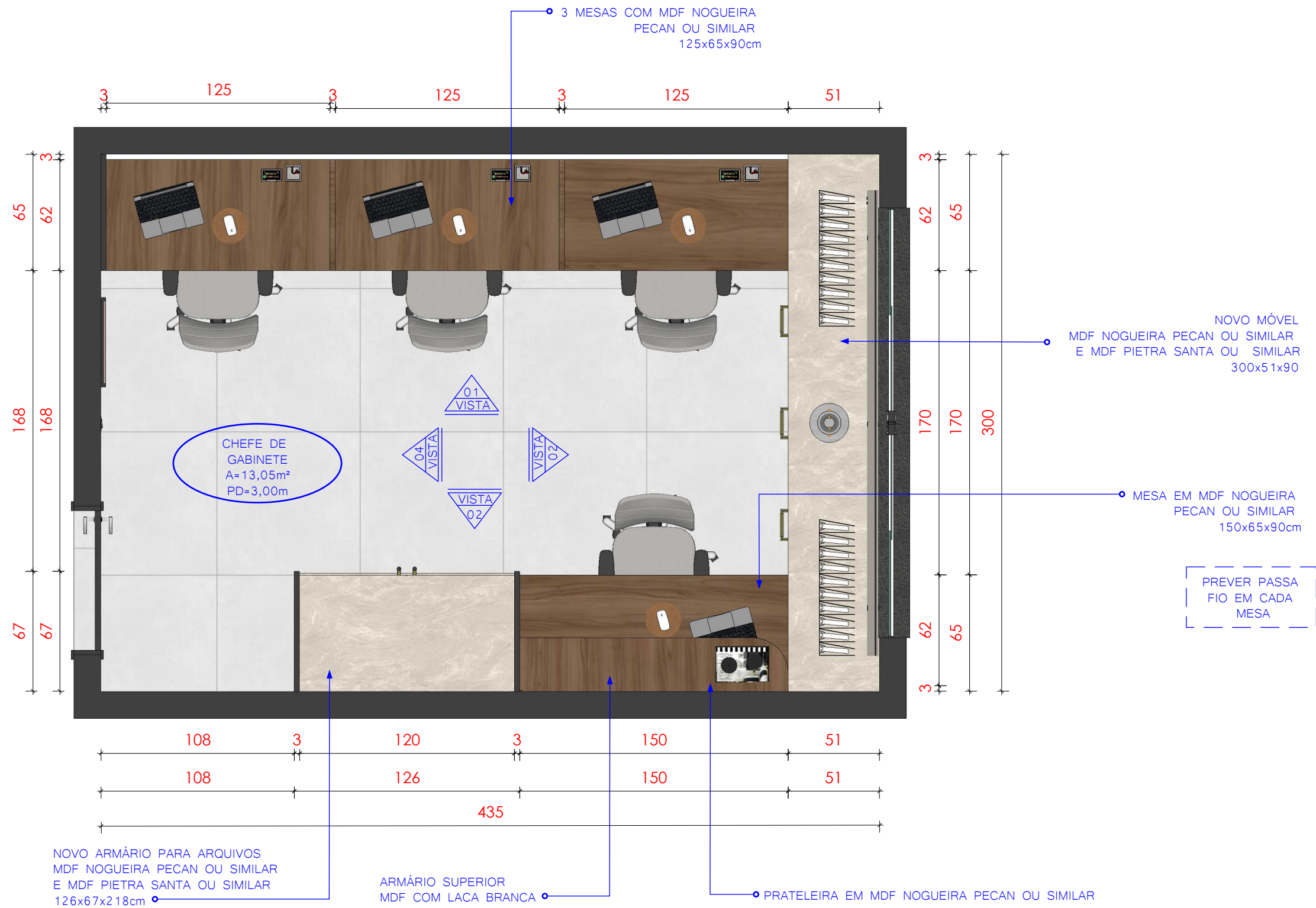
1 PLANTA DE LAYOUT_CHEFE DE GABINETE ESCALA 1:25
