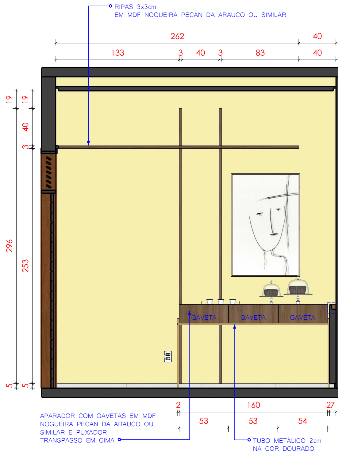
1 VISTA 01_SALA DE ESPERA ESCALA 1:25
