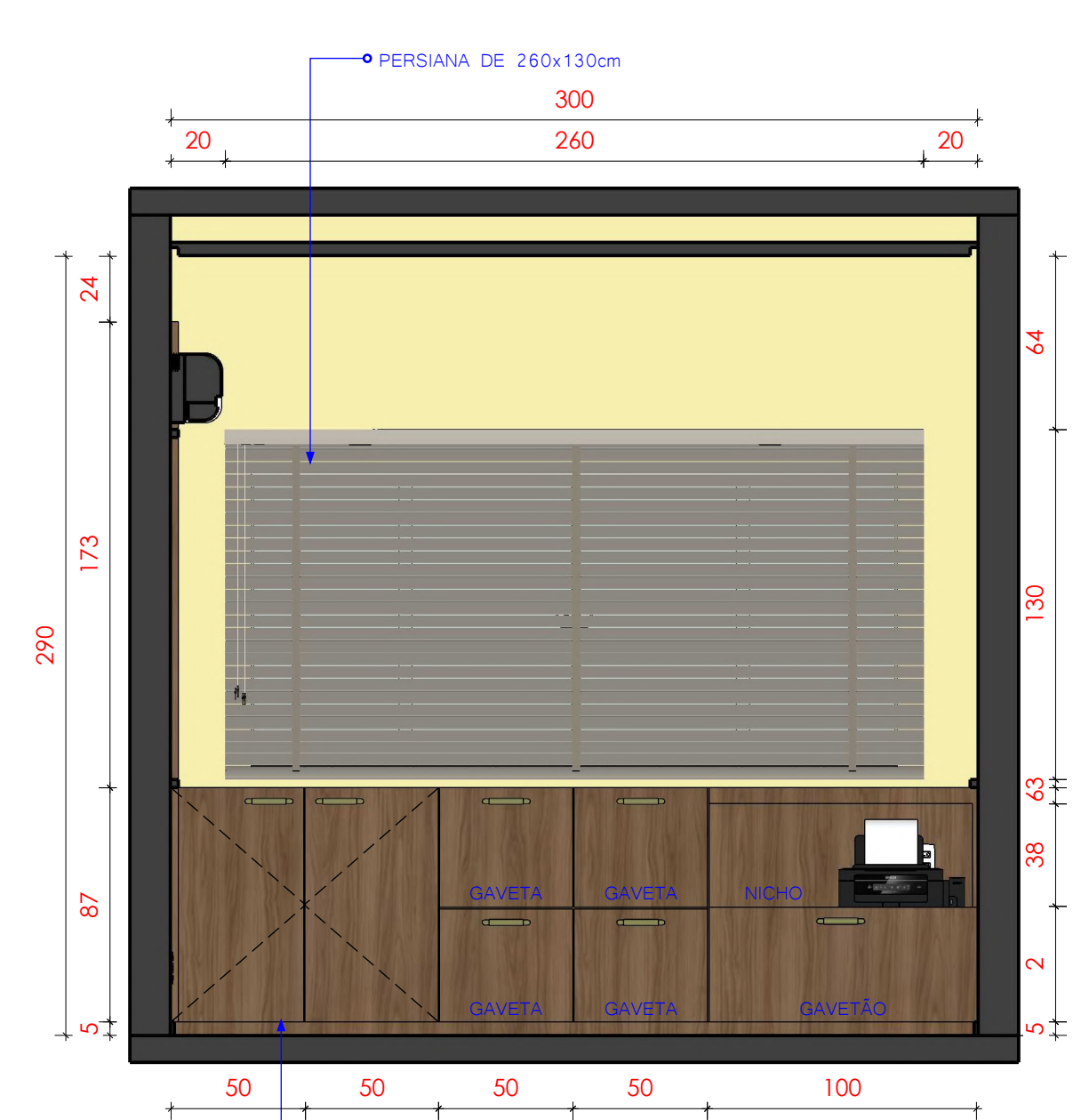
1 VISTA 01_SALA DE SUPLENTES ESCALA 1:25
