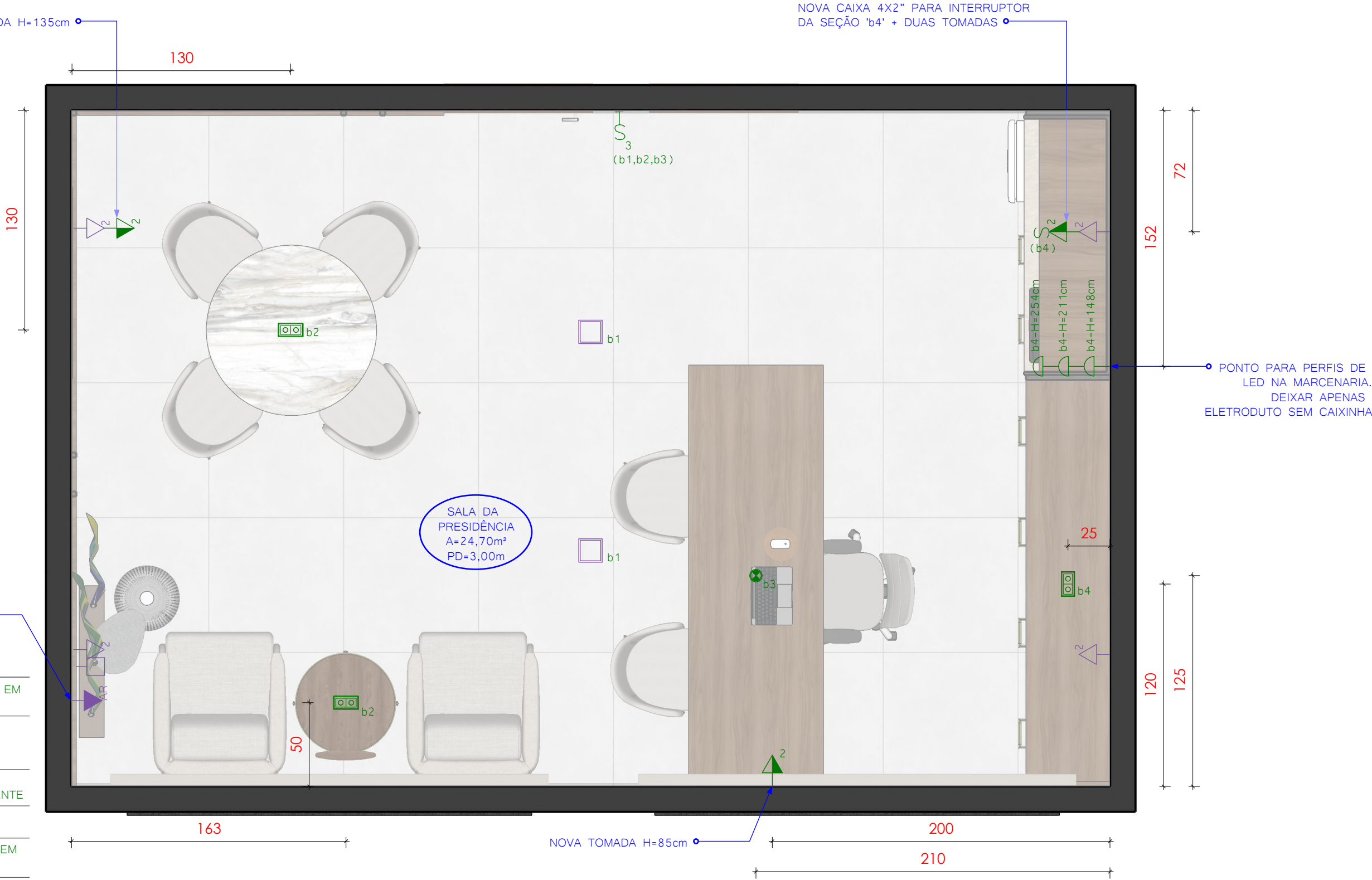
1 PLANTA DE PONTOS ELÉTRICOS E LUMINOTÉCNICOS_SALA DA PRESIDÊNCIA ESCALA 1:25
