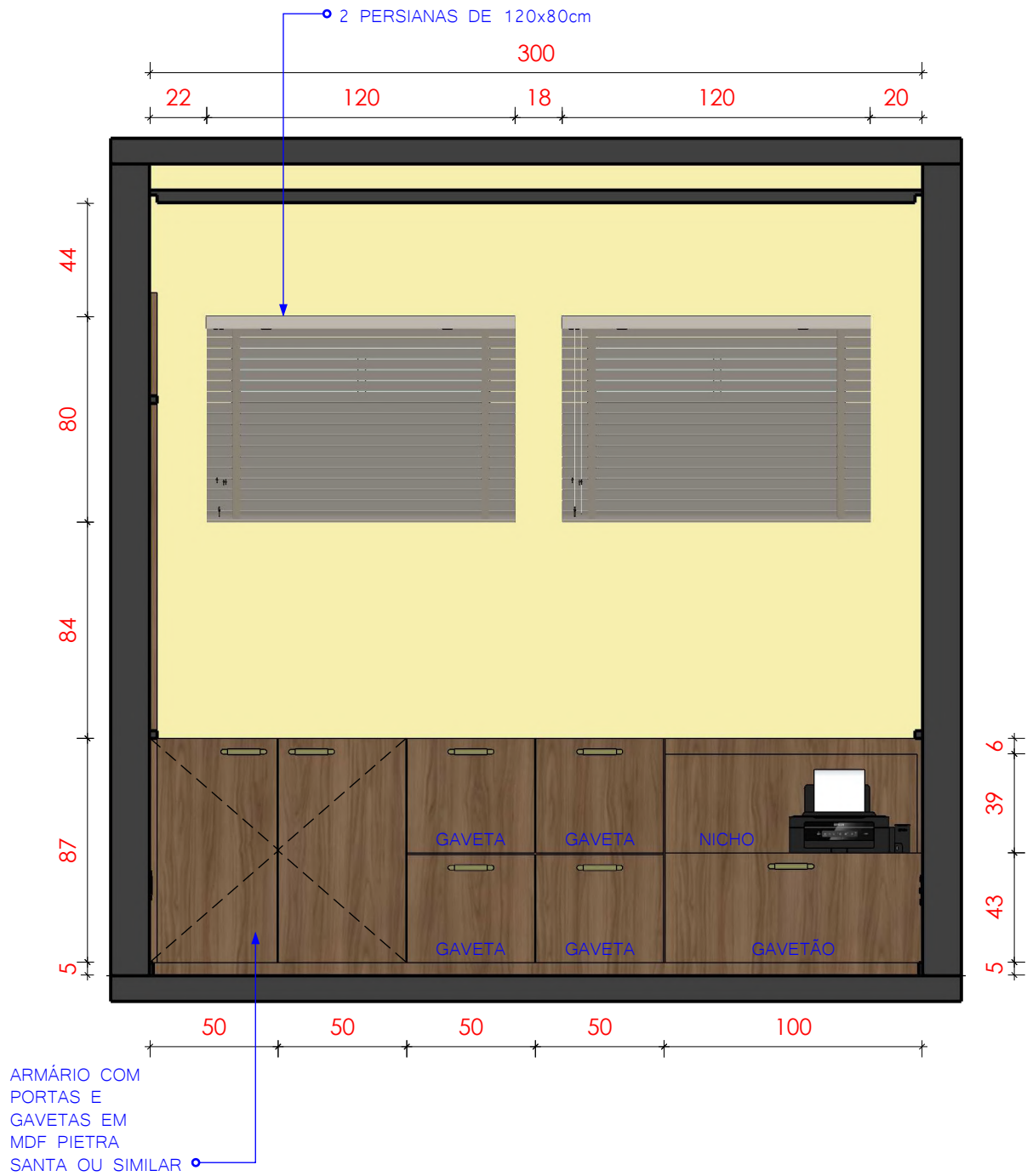
1 VISTA 01_SALA DE VEREADORES TIPO 1 ESCALA 1:25
