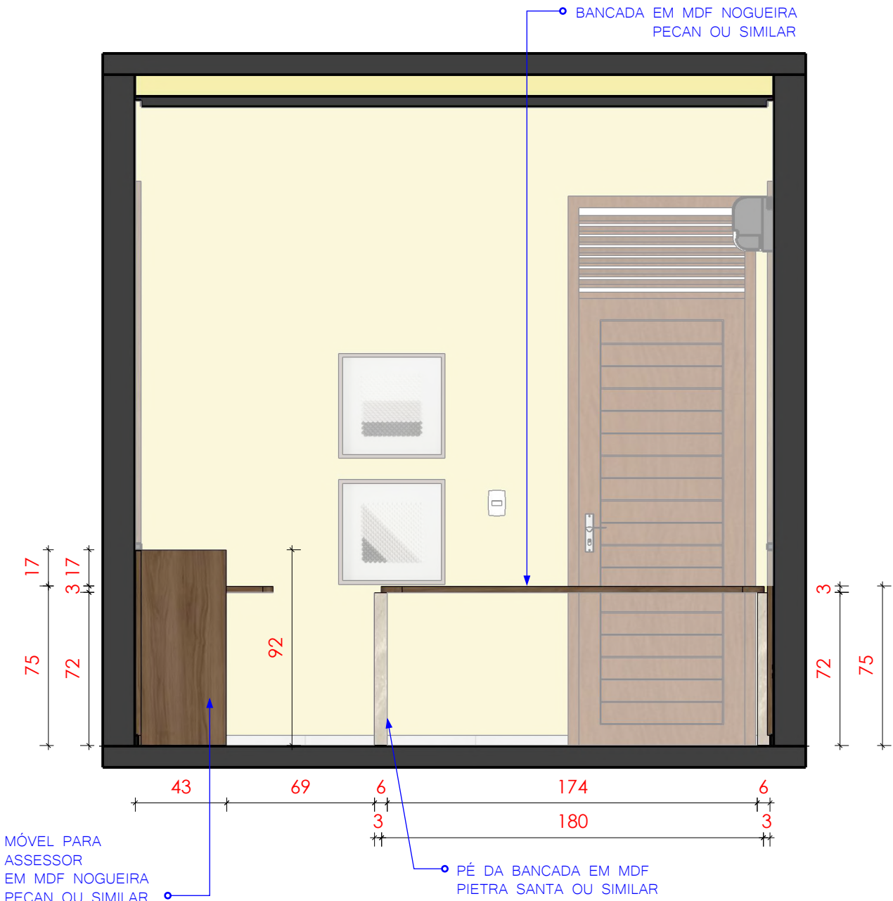
1 VISTA 03_SALA DE VEREADORES TIPO 2 ESCALA 1:25
