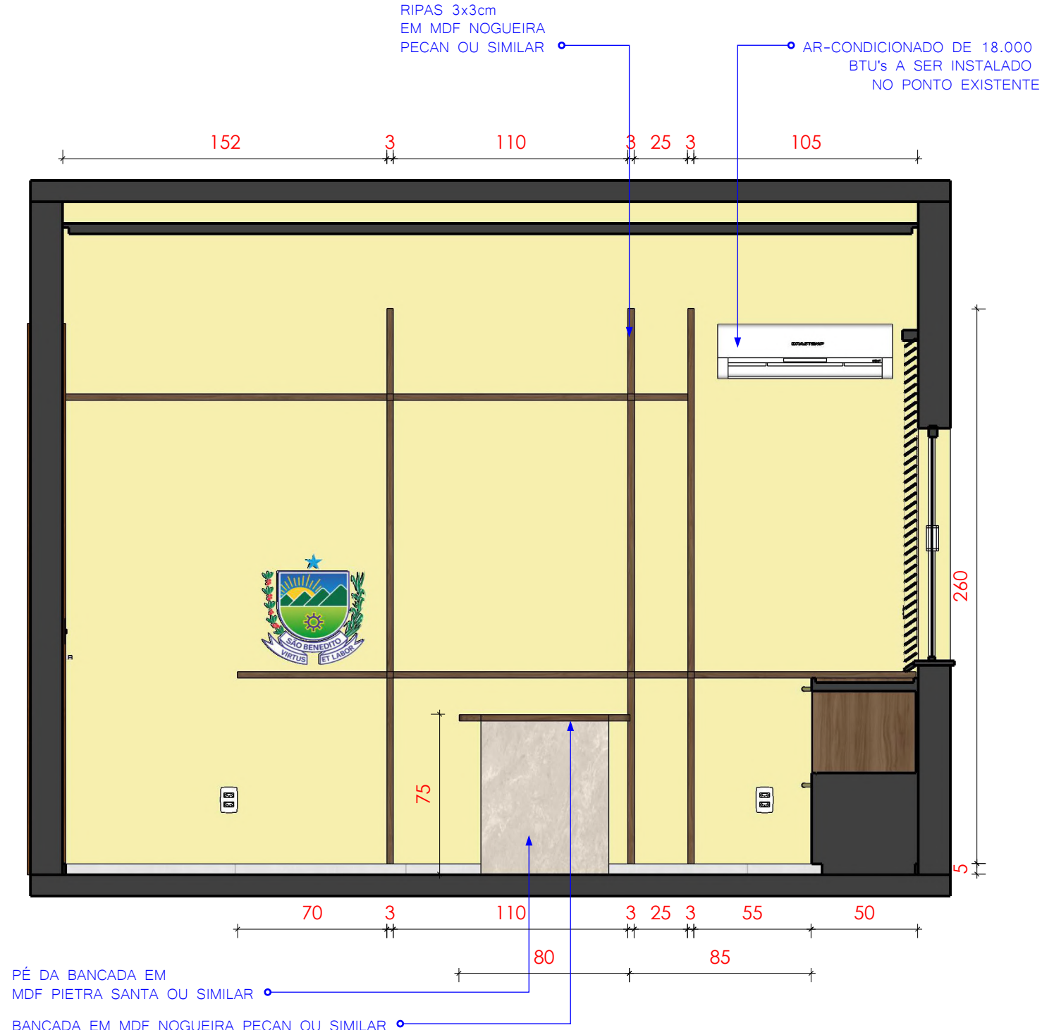
2 VISTA 04_SALA DE VEREADORES TIPO 2 ESCALA 1:25
