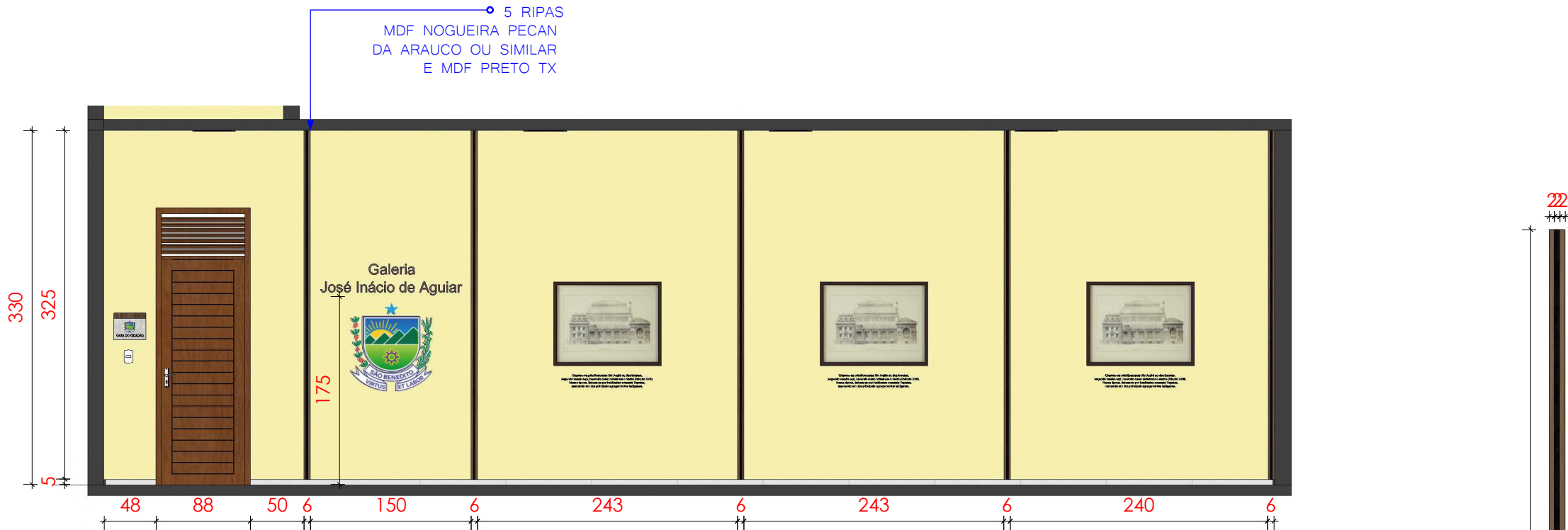
1 VISTA 01_MINI MUSEU ESCALA 1:50
