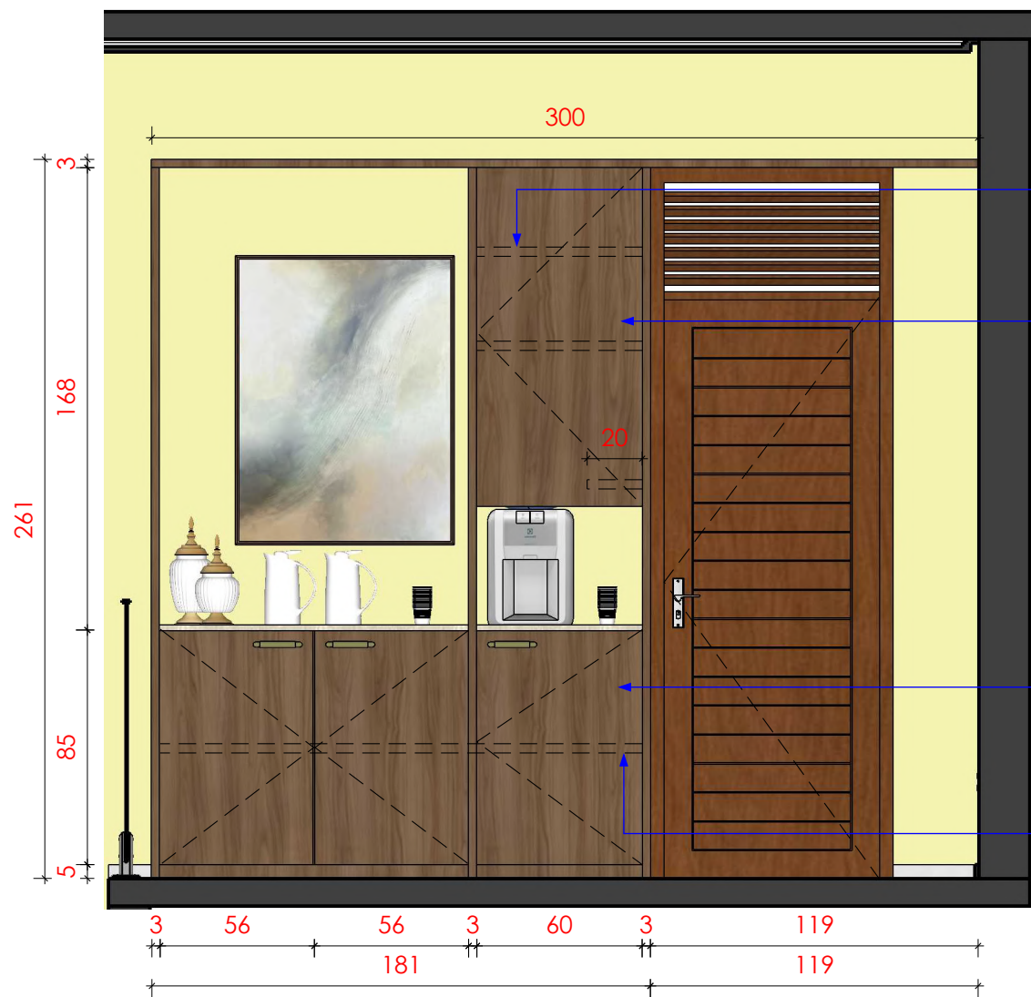
1 VISTA 04_RECEPÇÃO SUPERIOR ESCALA 1:25
