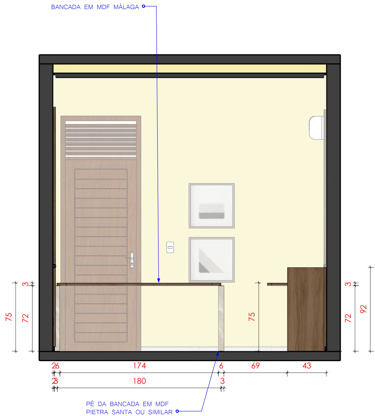
1 VISTA 03_SALA DE VEREADORES TIPO 1 ESCALA 1:25
