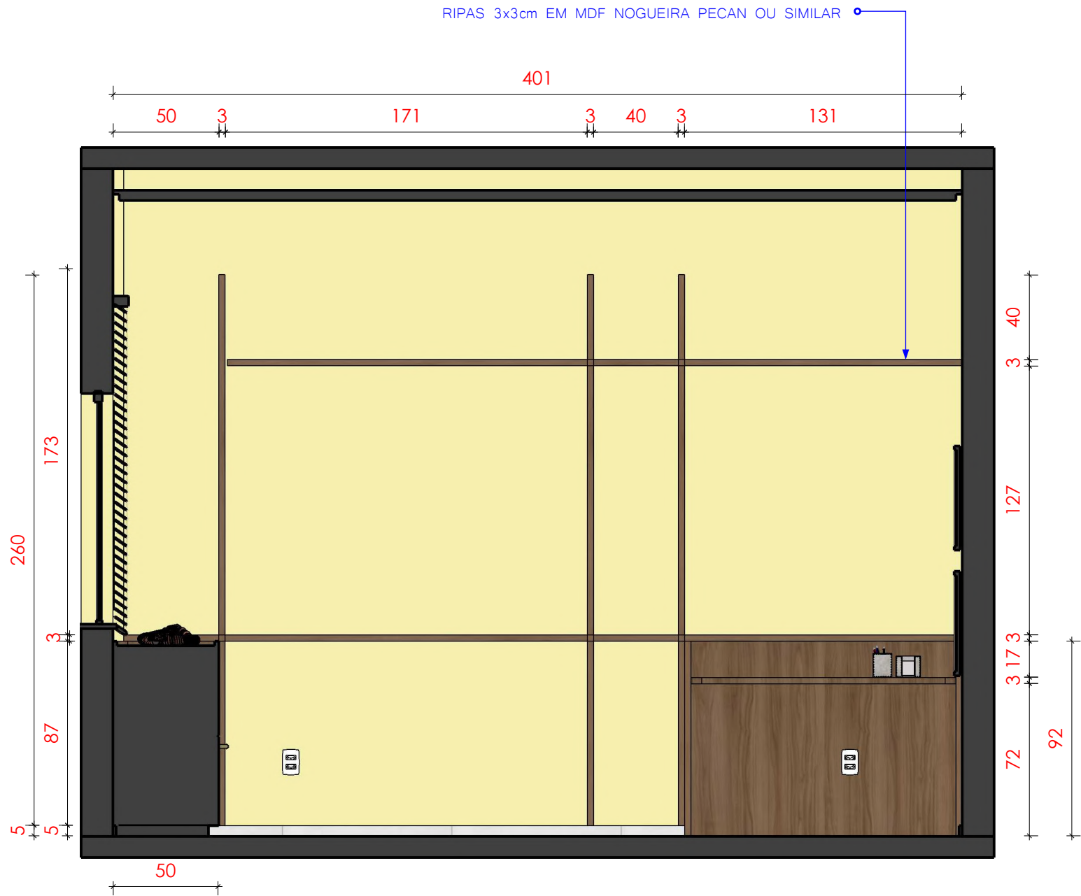
2 VISTA 02_SALA DE VEREADORES TIPO 2 ESCALA 1:25
