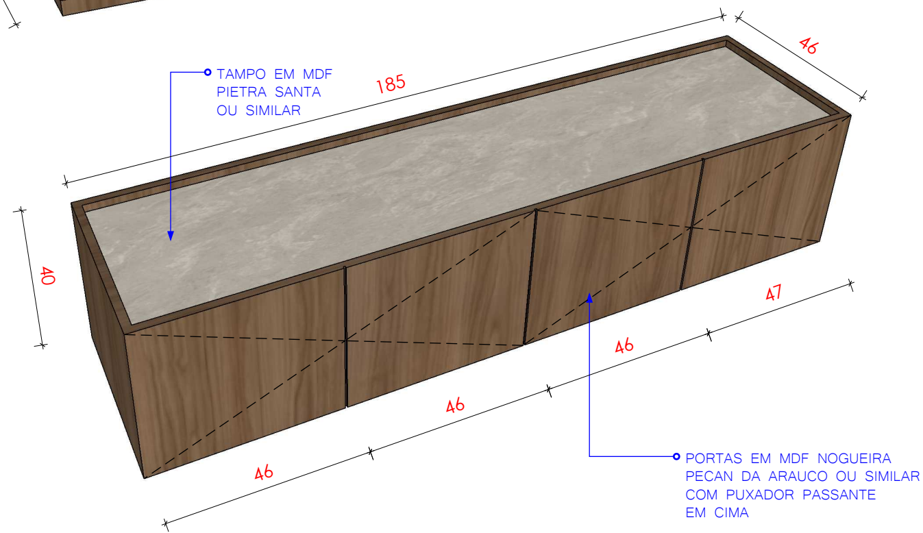
3 DETALHAMENTO 03_PROCURADORIA DA MULHER
