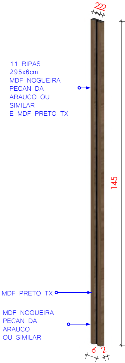
2 DET. RIPAS_SALA DE COMISSÕES ESCALA 1:10
