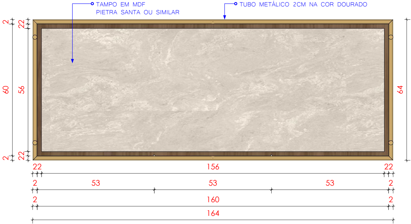
1 DETALHAMENTO APARADOR _SALA DE ESPERA ESCALA 1:10
