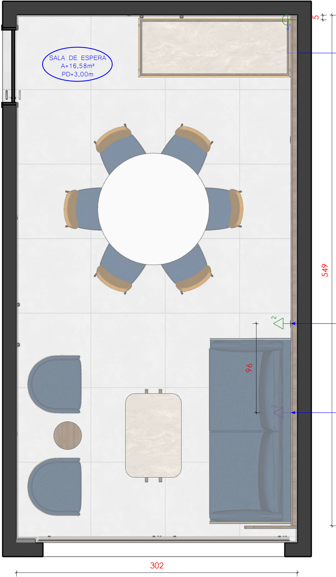
2 PLANTA DE PONTOS ELÉTRICOS E LUMINOTÉCNICO_SALA DE ESPERA ESCALA 1:25
