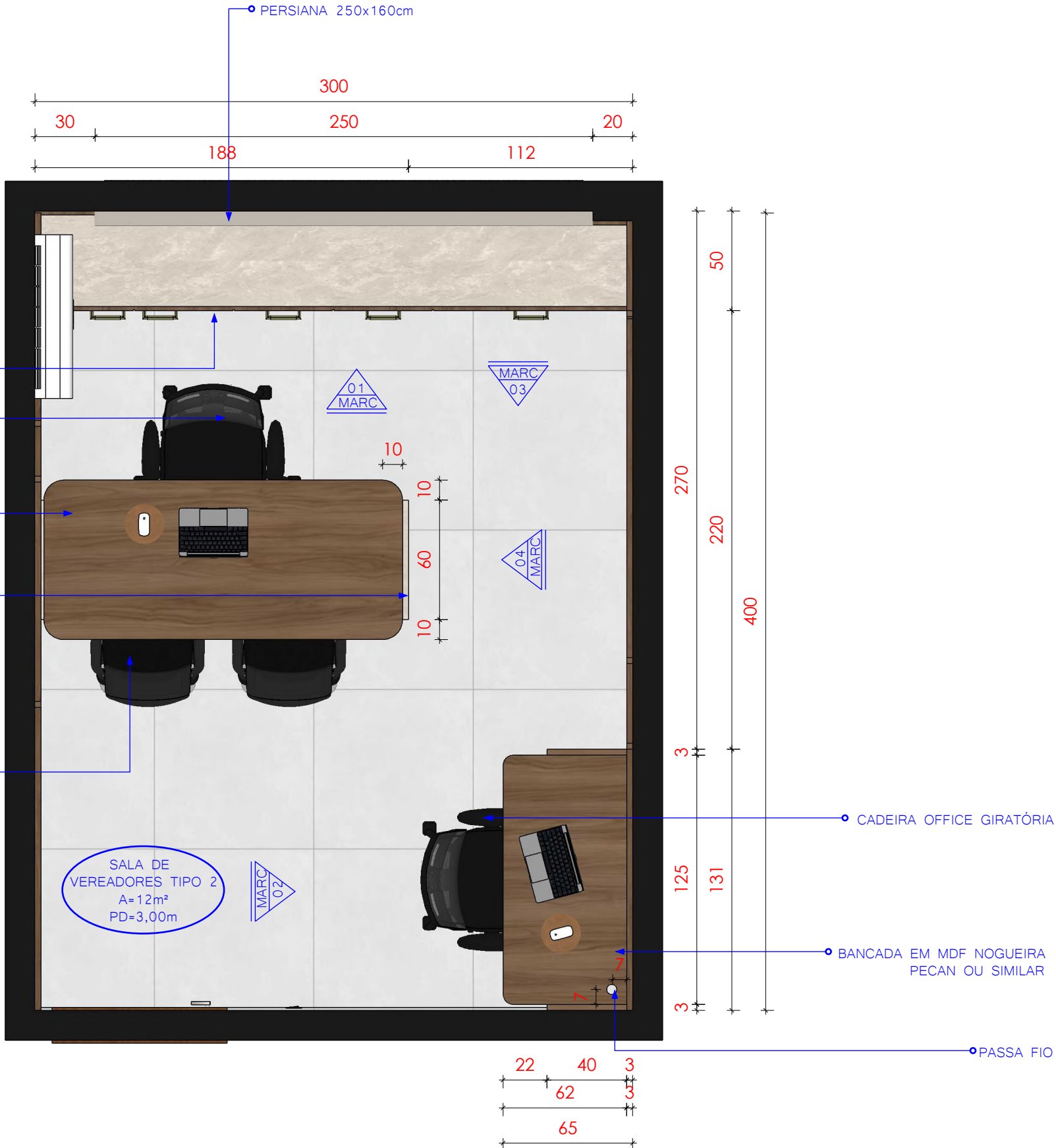
1 PLANTA DE LAYOUT_SALA DE VEREADORES TIPO 2 ESCALA 1:25
