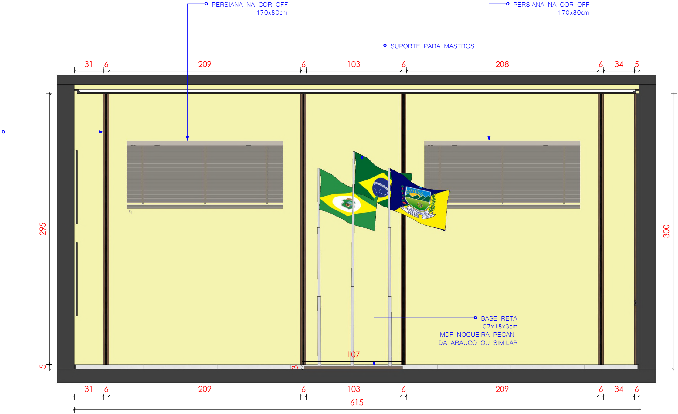
1 VISTA 02_SALA DE COMISSÕES ESCALA 1:25
