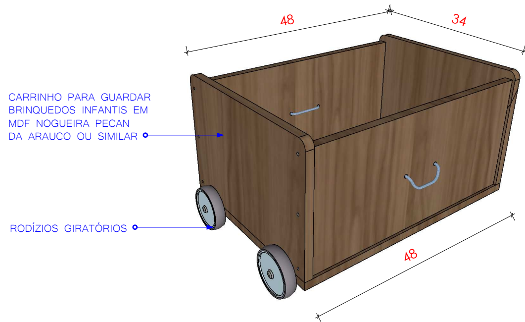
2 DETALHAMENTO 03_PROCURADORIA DA MULHER
