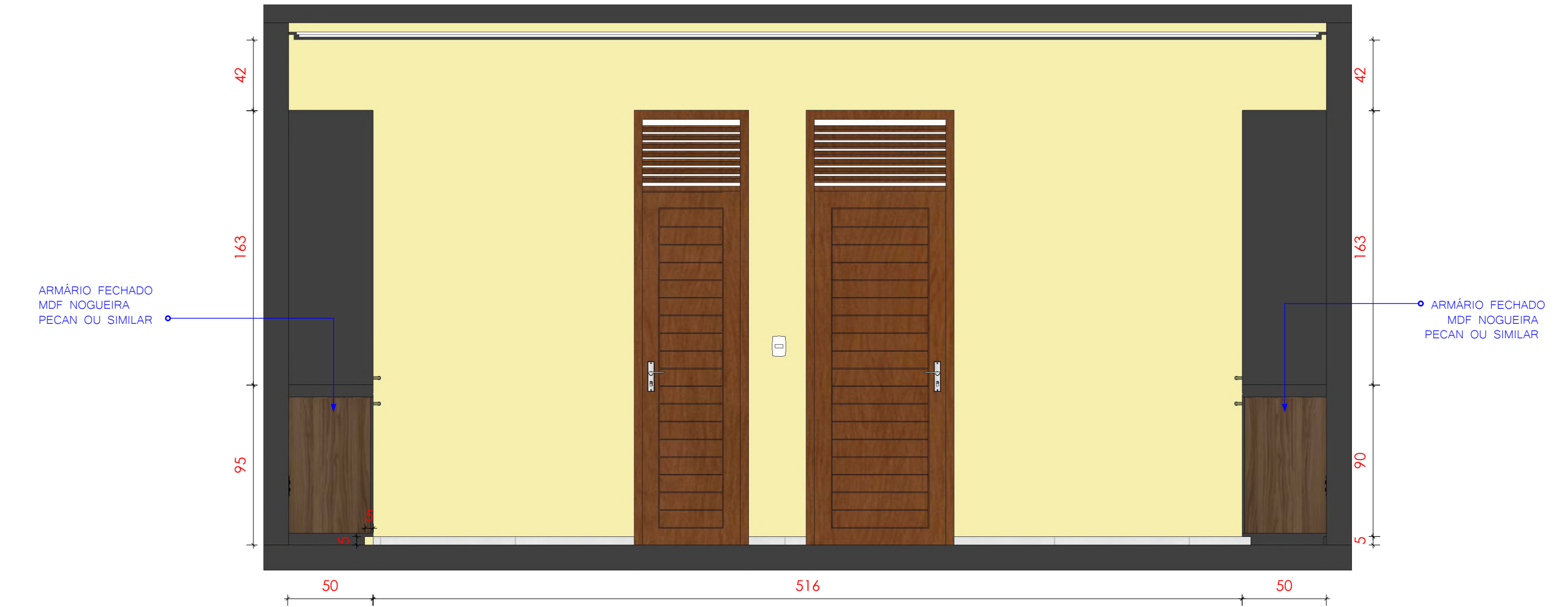
1 VISTA 04_CONTABILIDADE E LICITAÇÃO ESCALA 1:25
