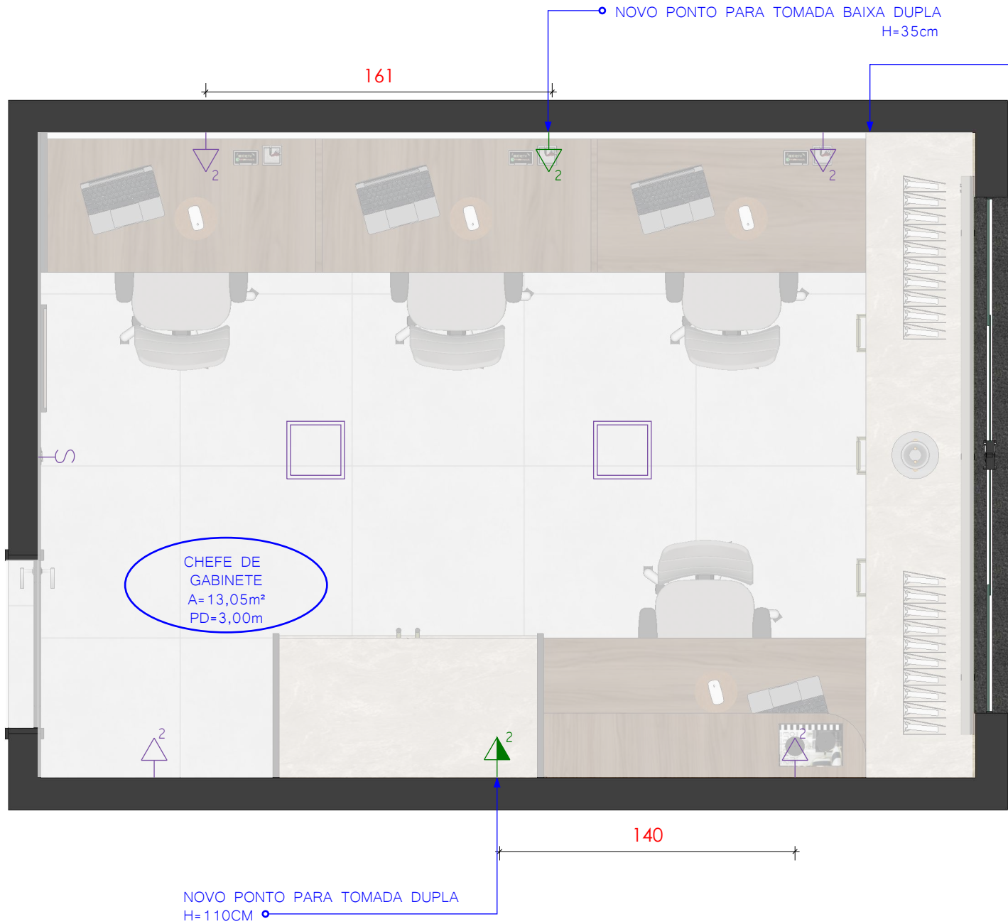
1 PLANTA PONTOS ELÉTRICOS E LUMINOTÉCNICOS_CHEFE DE GABINETE ESCALA 1:25
