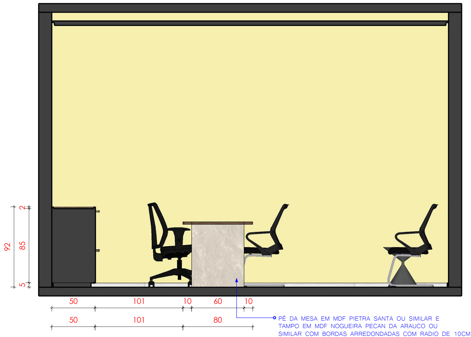
1 VISTA 02_SALAS A e B ESCALA 1:25
