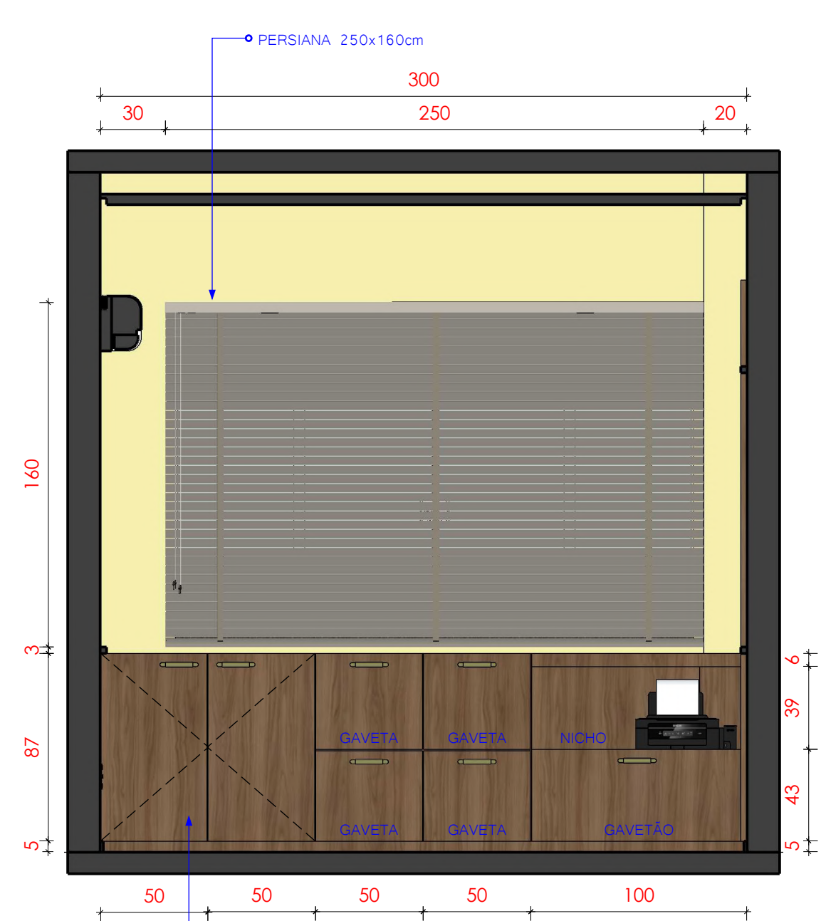
1 VISTA 01_SALA DE VEREADORES TIPO 2 ESCALA 1:25
