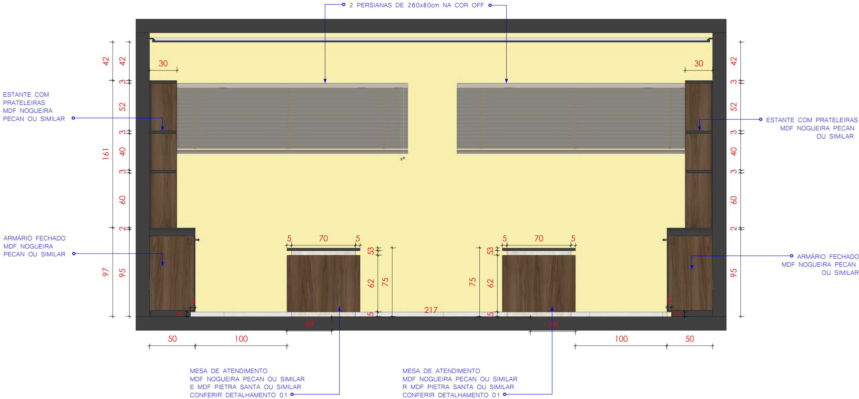
1 VISTA 03_CONTABILIDADE E LICITAÇÃO ESCALA 1:25
