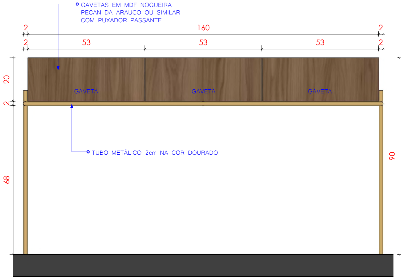
2 DETALHAMENTO APARADOR _SALA DE ESPERA ESCALA 1:10
